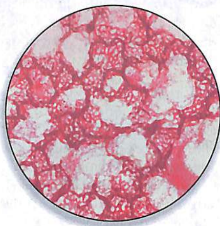
Альвеолы
