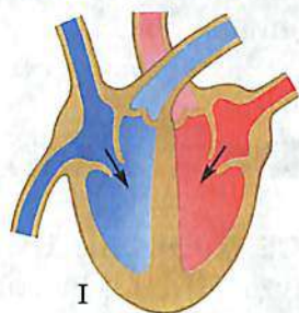
СЕРДЕЧНЫЙ ЦИКЛ
