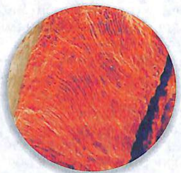
Дентин
