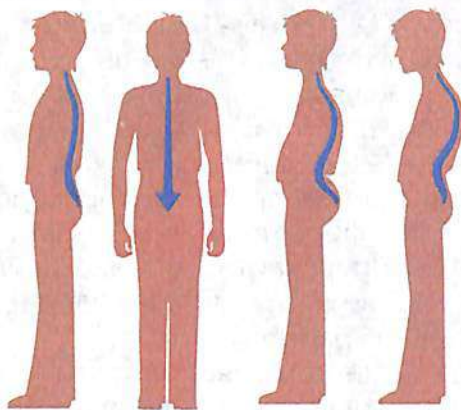
Правильная осанка
